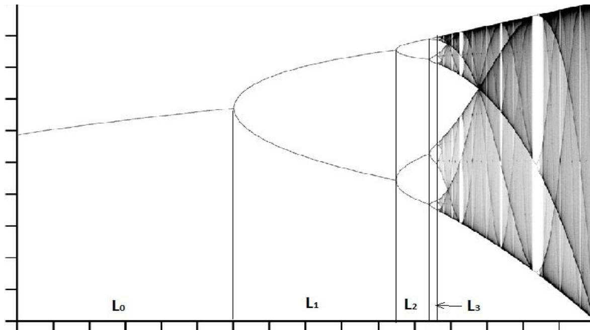
Рис. 1. Каскад бифуркаций с удвоением периода в сценарии перехода к хаосу Фейгенбаума.
